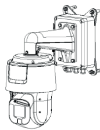
Montaje de cuello de cisne DS-1619ZJ
