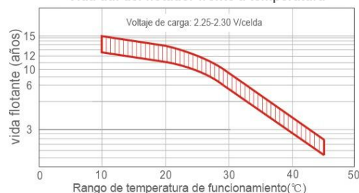
Vida útil del flotador frente a temperatura
