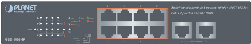
Figura 2-1: Panel frontal del conmutador GSD-1008HP
