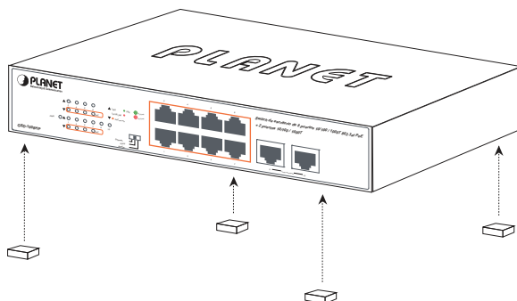
Figura 3-1: Colocación de los pies de goma en el GSD-1008HP
