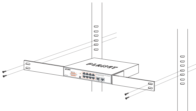
Figura 3-3: Montaje del GSD-1008HP en un bastidor
