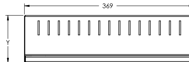
VISTA LATERAL
