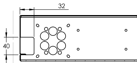
VISTA POSTERIOR
