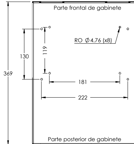
VISTA INFERIOR
