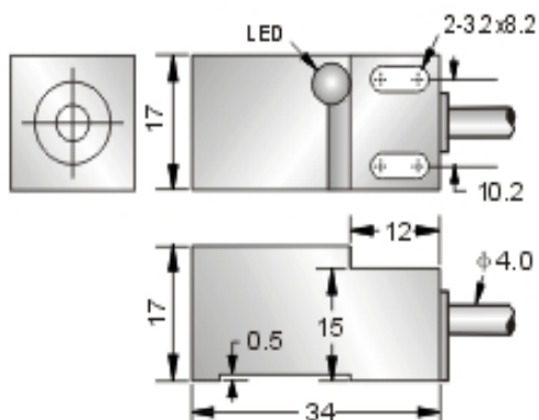
Dimensiones (mm)
