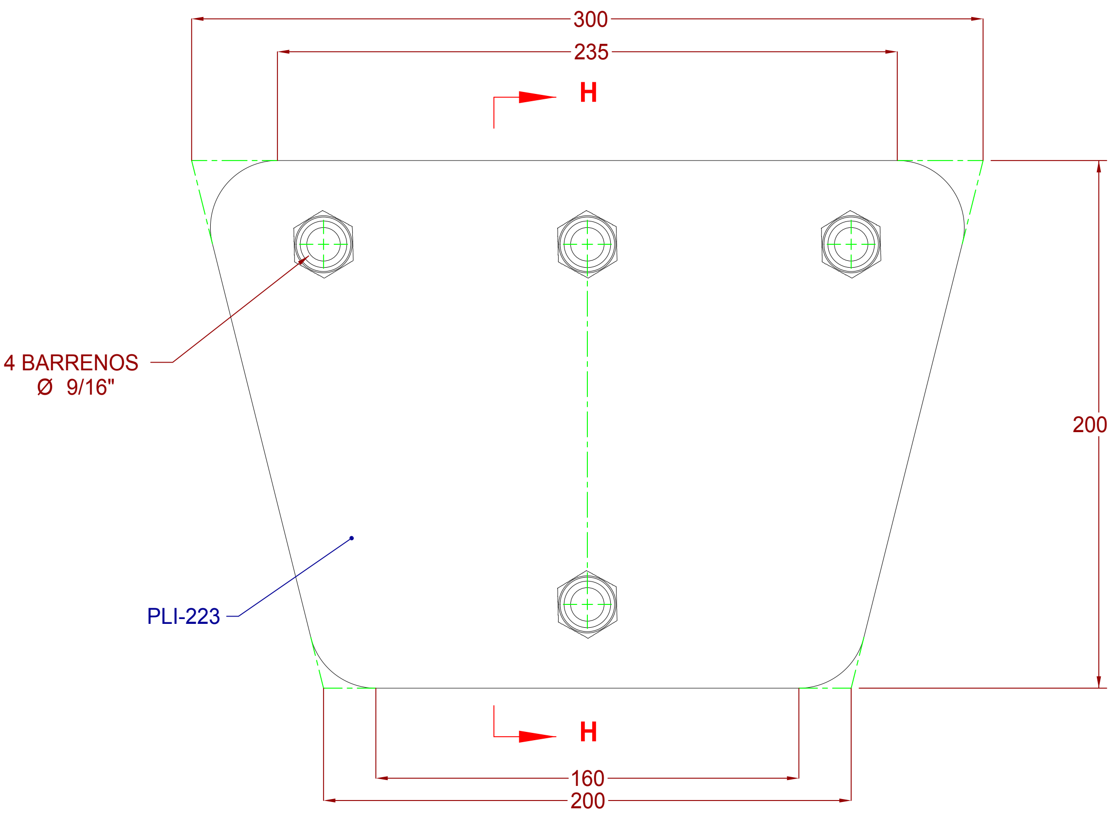
DETALLE DE ARMADO PLACAS IGUALADORAS SJTP3G (20-20-30)
