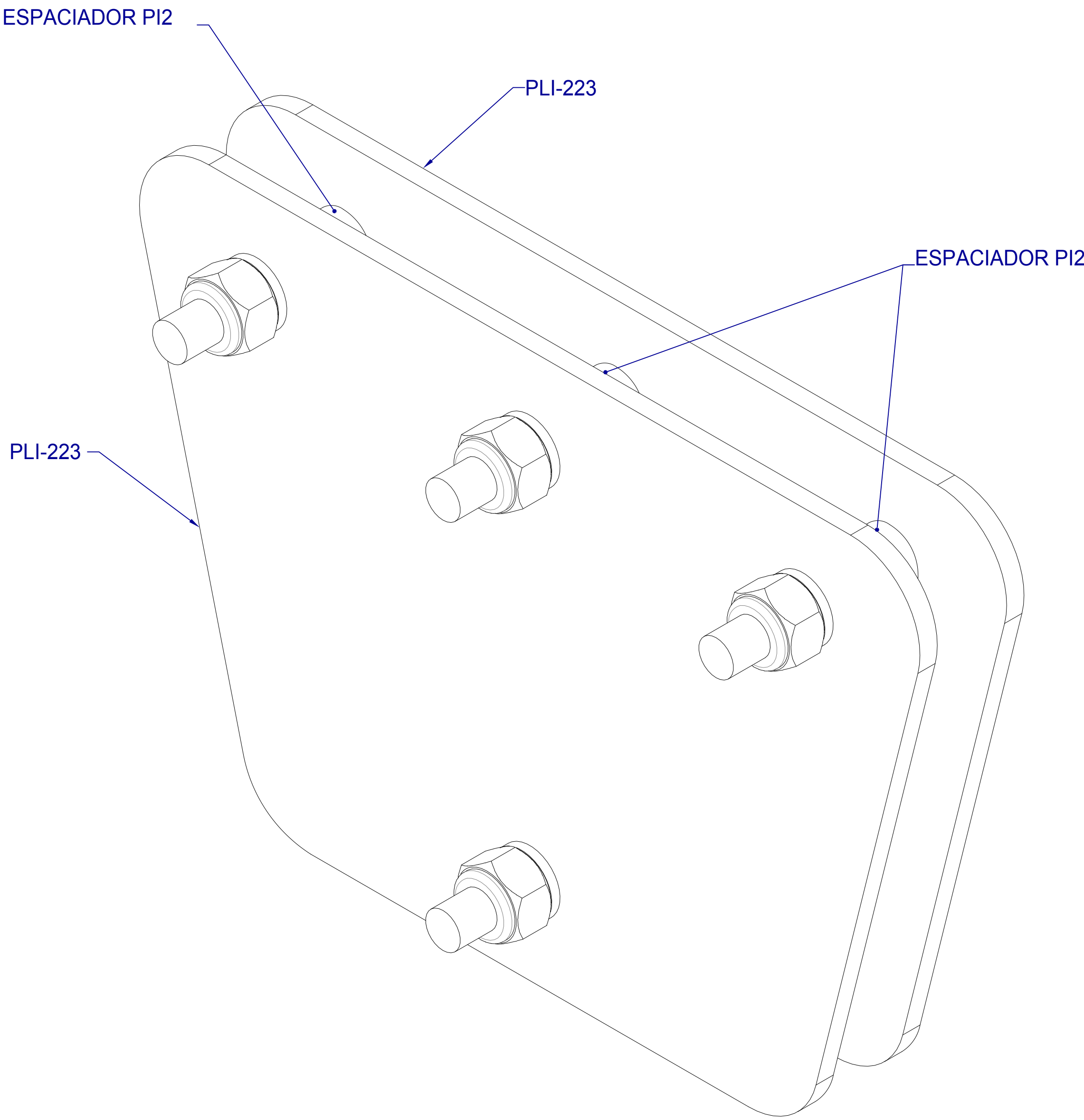
VISTA ISOMÉTRICA PLACAS IGUALADORAS SJTP3G (20-20-30)
