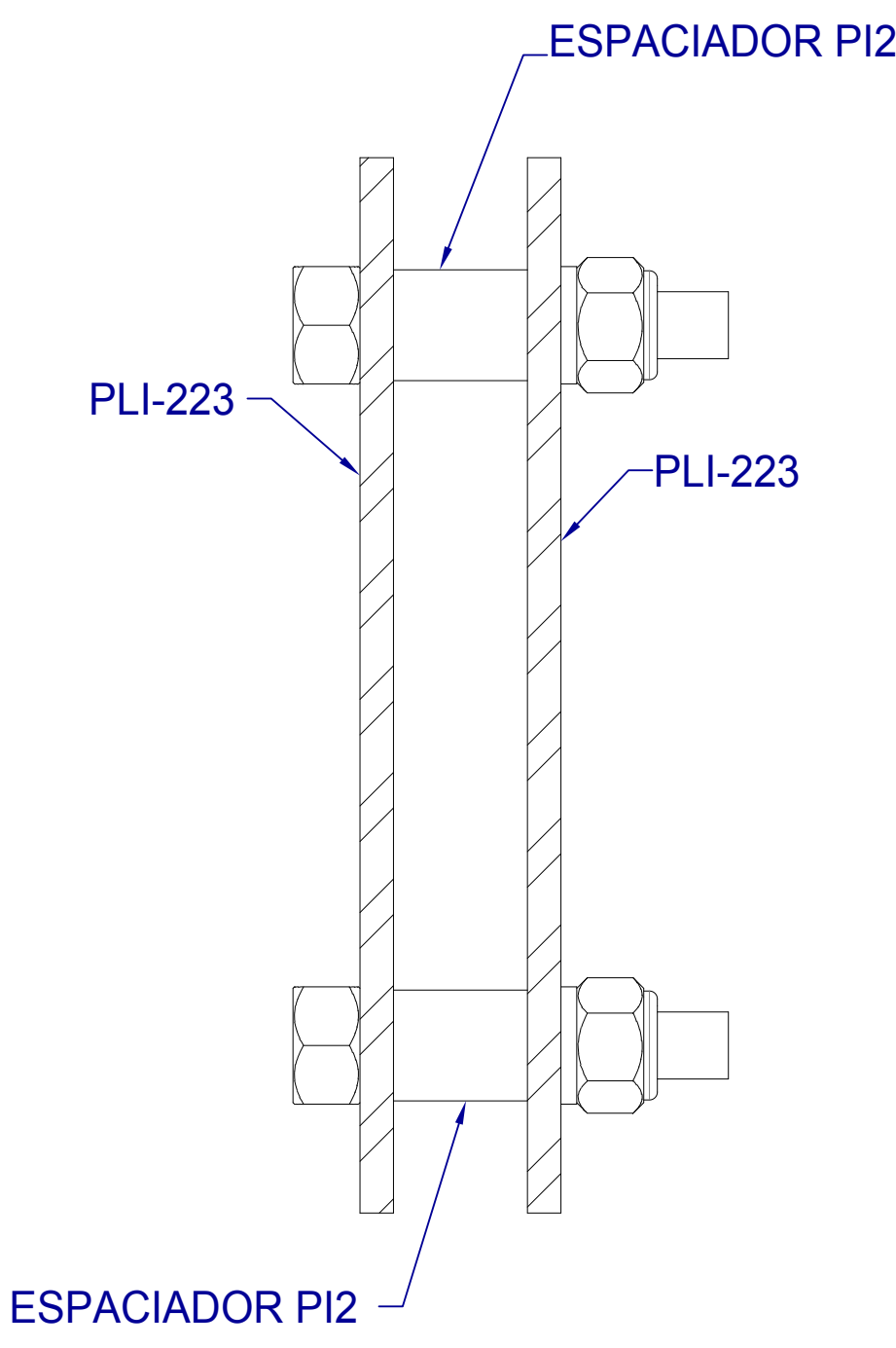
SECCIÓN H-H ESCALA 1 : 1.5
